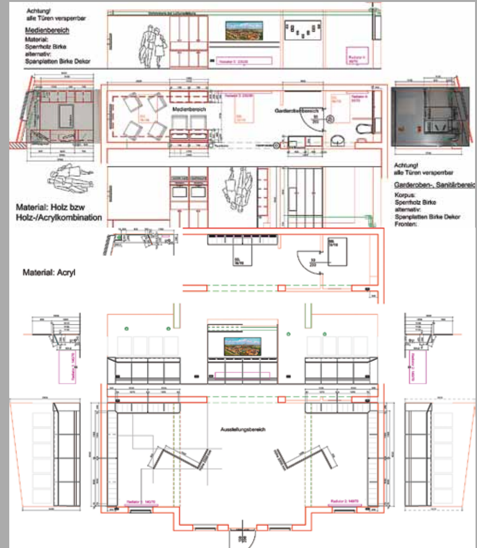
Einrichtungsplan Museum Marienthal (Medienbereich, Sanitärbereich und Ausstellungsbereich).
